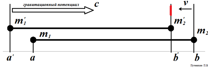
Рис.5. Масса в конце движущегося стержня испытывает силу, как если бы длина стержня была меньше исходной
